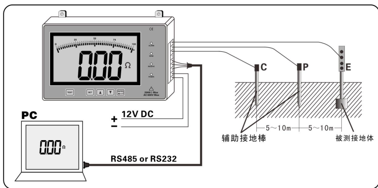
图 3（安装连接示意图）
