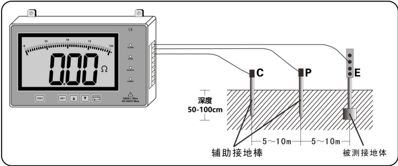
图 2（测量单点接地示意图）
