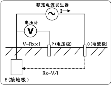
图 1（测量原理图）
