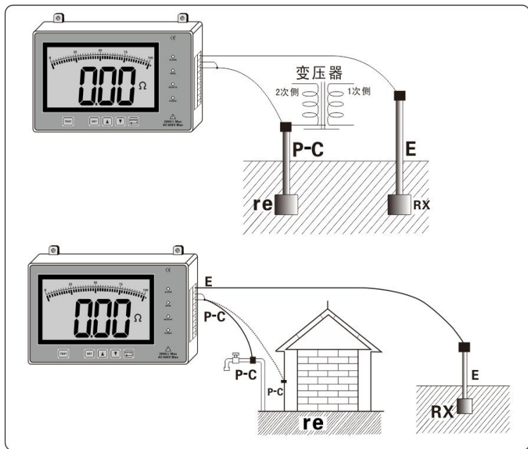
图 4（简易二线法测试接线示意图）
